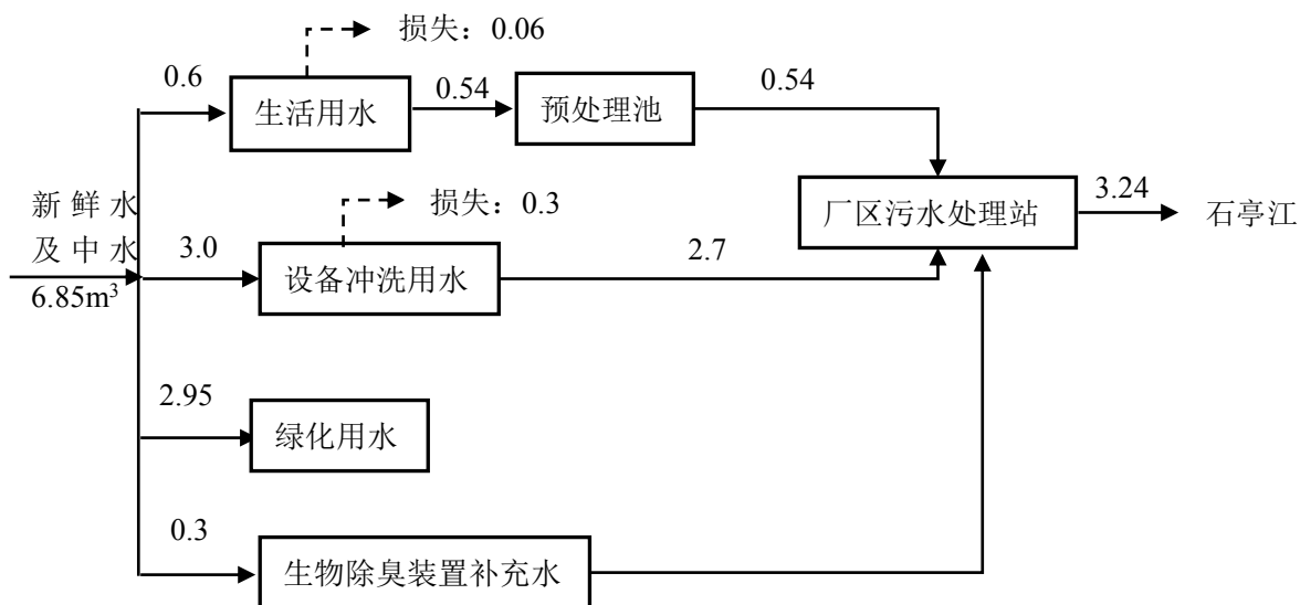
图 3-1 项目总用水量平衡图 m^3/d
