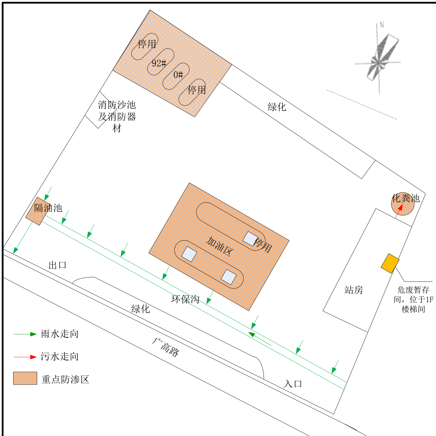
附图2 项目总平面布置图
