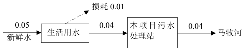
图 2-1 本项目水平衡图 (m 3 /d)
