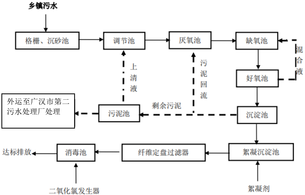
图 2-2 污水处理站工艺流程图
